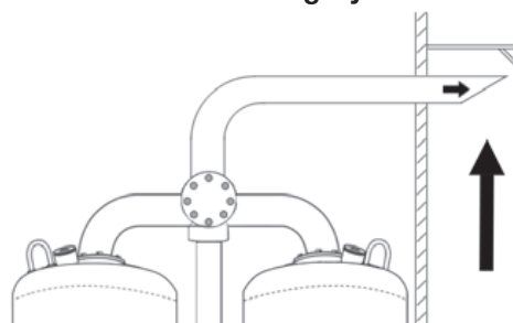
Osłona atmosferyczna przy bocznym ułożeniu przewodu
